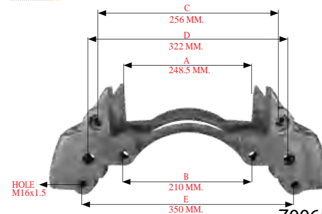
221 90 105 > BALATA TAŞIYICI / CARRIER
