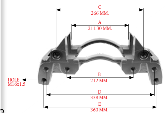
2219 0107 > BALATA TAŞIYICI / CARRIER
