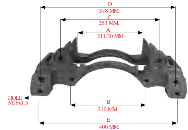
2229 0104 > BALATA TAŞIYICI 22.5" CARRIER - L - 22.5"
