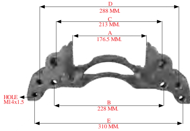
222 90101 > BALATA TAŞIYICI 17.5" CARRIER - R - 17.5"
