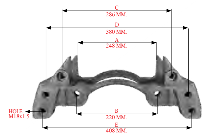
221 90 104 > BALATA TAŞIYICI / CARRIER
