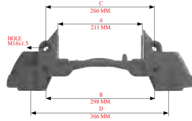
2219 0101 > BALATA TAŞIYICI / CARRIER
