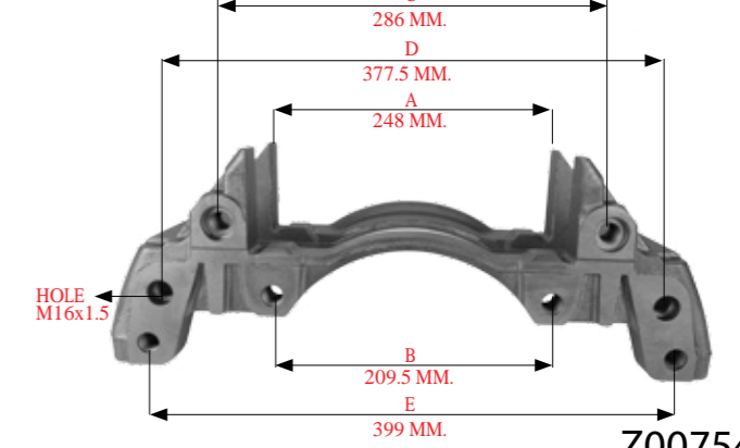
221 90 102 > BALATA TAŞIYICI / CARRIER
