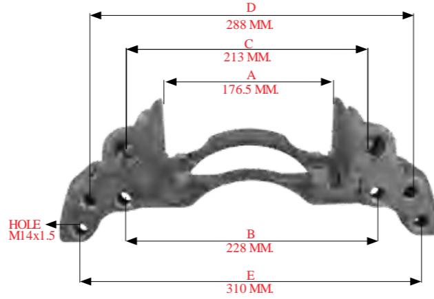
222 90102 > BALATA TAŞIYICI 17.5" CARRIER - L - 17.5"
