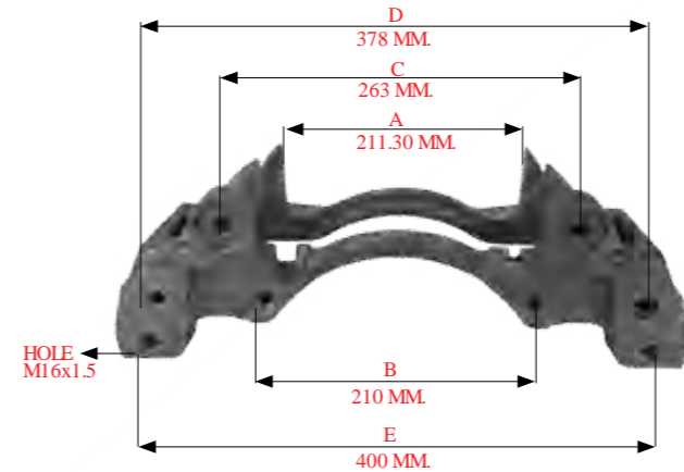
222 90103 > BALATA TAŞIYICI 22.5" CARRIER - R - 22.5"
