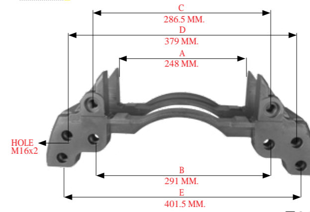
2219 0103 > BALATA TAŞIYICI / CARRIER
